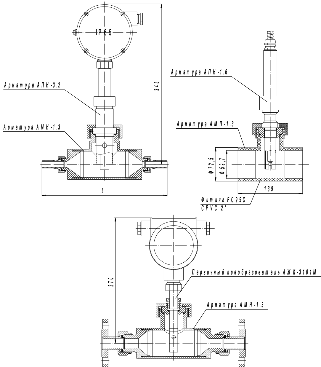
Рисунок 3 Примеры использования арматур магистральных АМН-1.3; АМП-1.3
