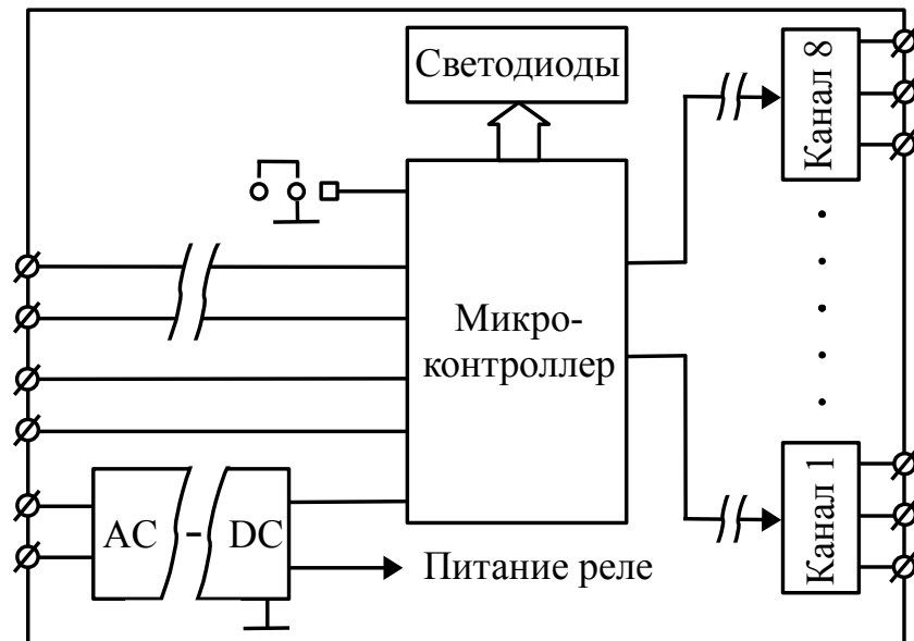
Рисунок 2 - Функциональная схема БВД-8.2
